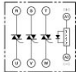
G3PB-□□□B-2N-VD
