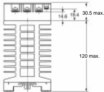
G3PB-□□□B-2N-VD
